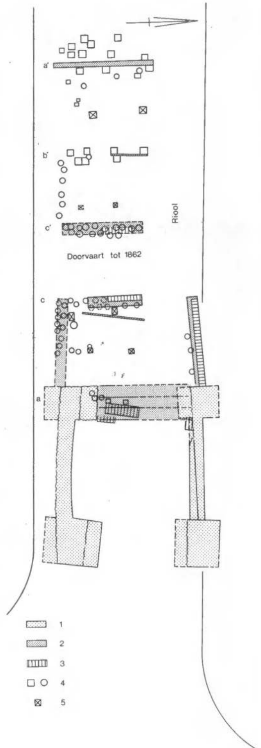
Afb. 1. Veldpoort en veldbrug, schaal 1 : 150. Opmeting Openbare Werken Enschede (G. v.d. Ziel). Legenda - 1 : metselwerk van de poort; 2: houten planken, balken, schotten; 3: blokken Bentheimer steen; 4: palen voor funderingen en beschoeiingen; 5: (wrs.) dragende palen van de brug.
