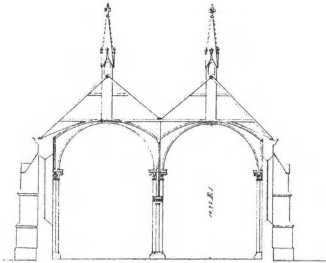
Fig. 2. Enschede, Grote Kerk. Dwarsdoorsnede (herbouwplan B. Looman 1862).
