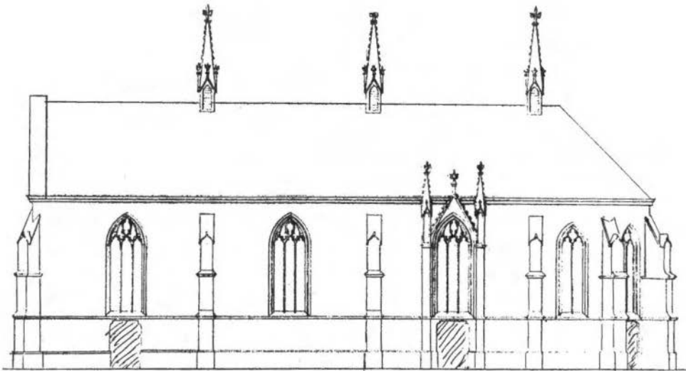
Fig. 1. Enschede, Grote Kerk. Zuidgevel (herbouwplan B. Looman 1862).
