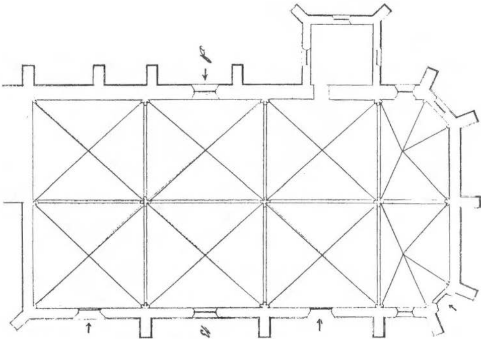
Fig. 3. Enschede, Grote Kerk. Plattegrond (herbouwplan B. Looman 1862).
