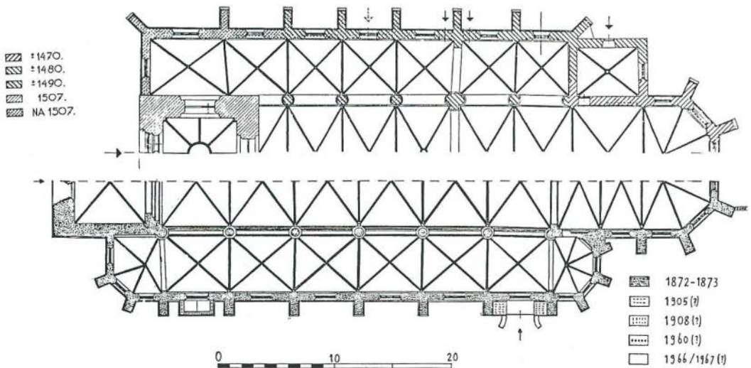
Plattegronden van de Ned. Herv. kerk te Winterswijk (bovenste helft) en van de R.K. in Delden (onderste helft) op dezelfde schaal getekend.
