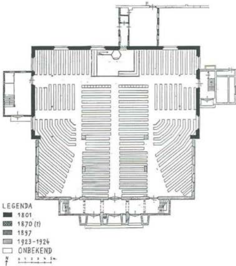
Afb. 4. Plattegrond van de Grote Kerk vóór 1966 (opmeting ir. T. van Hogeveest Amersfoort).
