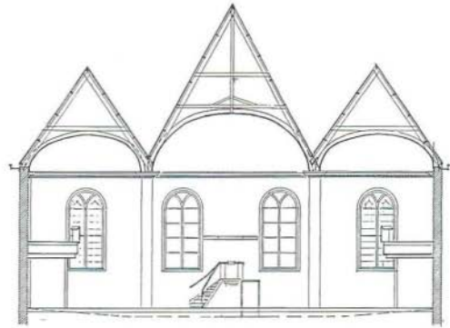
Afb. 5. Dwarsdoorsnede over de voorbouw van 1923-1924 (opmeting ir. T. van Hogeveest Amersfoort).
