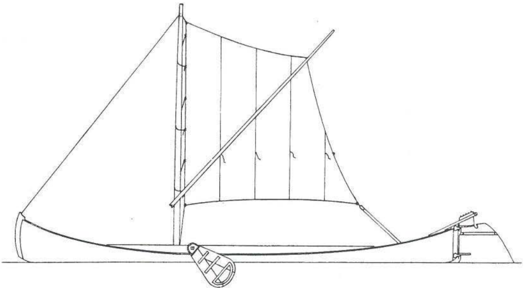
Zeilplan Vriezenveens turfschuitje: zeiloppervlak 8,5 m 2 . Met toestemming overgenomen uit: G.J. Schutte, Varen waar geen water is Hengelo (Ov), 1981, pag. 185.
