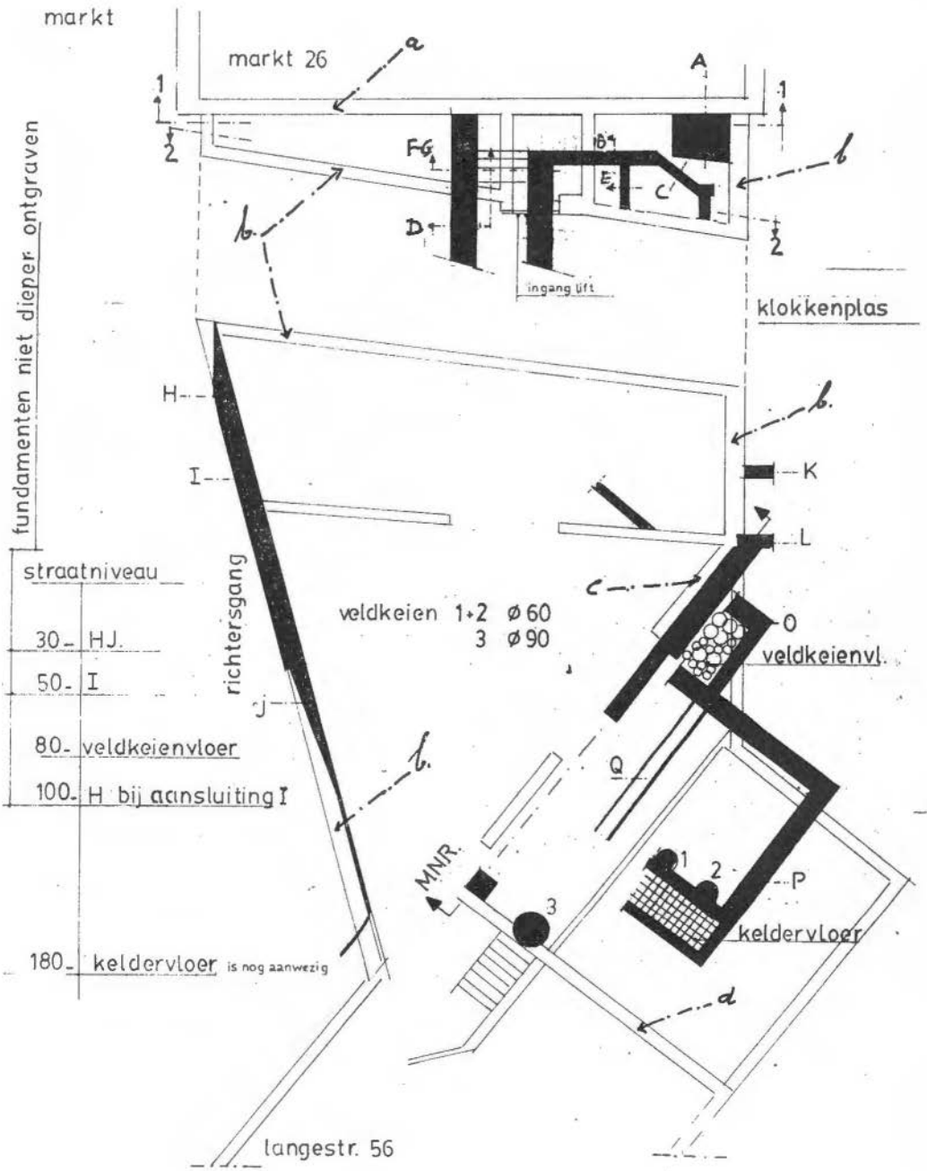
Tekening 2
