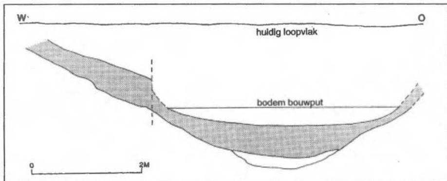
Oldenzaal-stadhuis oostzijde. Samengesteld, oostwestlopend dwarsprofiel over een omstreeks 1300 gedempte gracht (2,5 m diep) om de voorburcht? Gerasterde laag = gemengd zavelige grachttopvulling. Bij de verticale streepjeslijn sluiten de 2 profielen op elkaar aan. Schaal 1 : 80.
