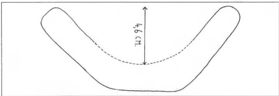
fig. 9: Dwarsdoorsnede van dakpan fig. 8. Het geglazuurde gootje is gearceerd.
