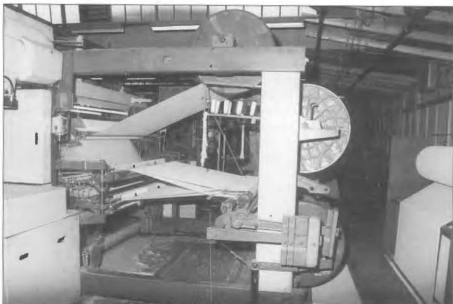
Weefmachine. Met verschillende rollen voor de pool- bind- en grondkettingdraden. FOTO: H. PASKAMP
