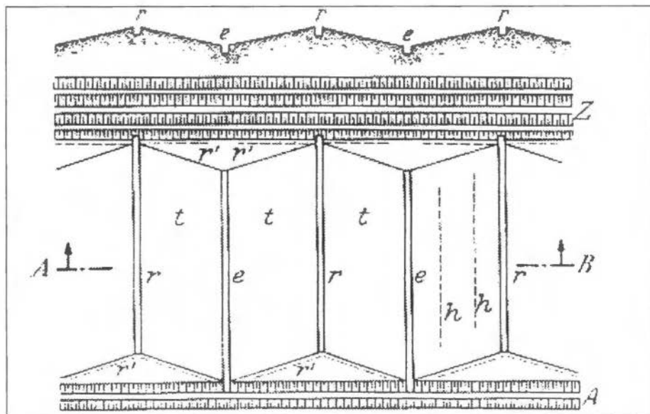
Figuur 2. Schematisch zij- en bovenaanzicht van een Rugbouwstelsel. Z = Aanvoerkanaal, r = aanvoerkanaaltje over rug, e = afvoerkanaal door lage deel, A = waterafvoerkanaal. r' = hellingshoek, met aan bovenzijde doorsnede A/B (uit: Schroeder, 1937).
