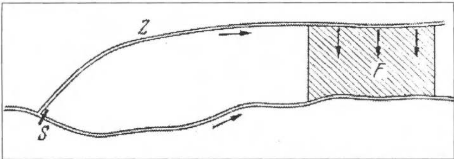
Figuur 1. Schematisch bovenaanzicht van een wilde bevoeiing. S = Stuw, Z = wateraanvoer, F = Vloeisloot (uit: Schroeder, 1937).
